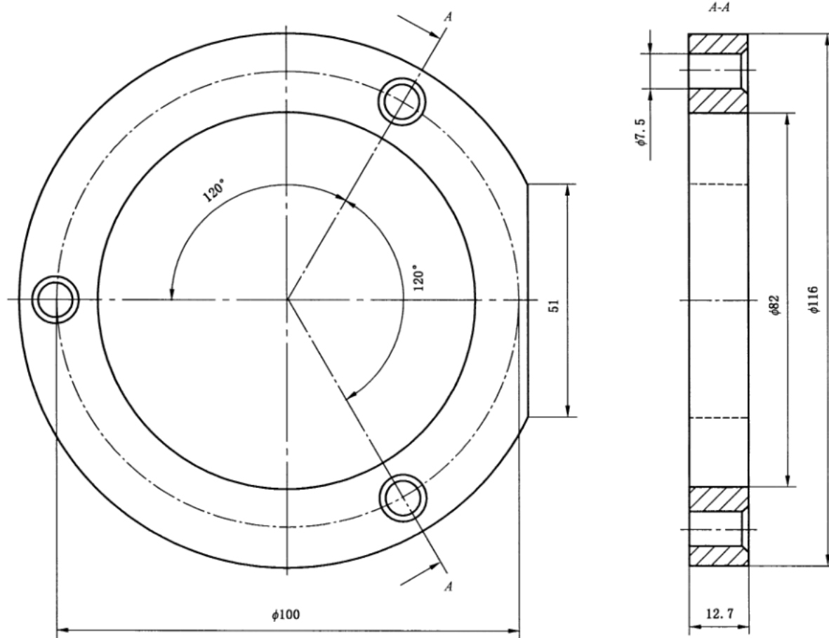
图 A.4 烧瓶定位环(耐火材料板)
