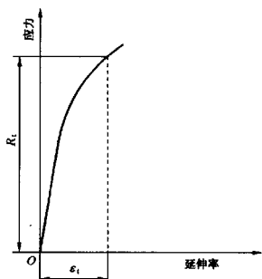
图4 规定总延伸强度( R_t )
