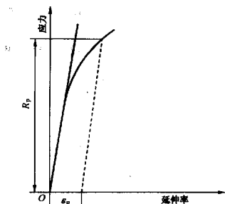
图3 规定非比例延伸强度( R_p )
