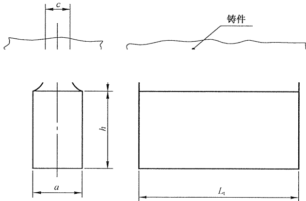
图 4 附铸试块
