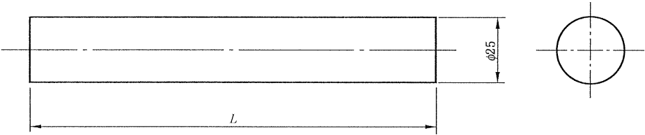
a) 试棒最小长度 L=150\text{ mm}
