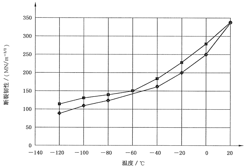
图 D.1 铁素体球墨铸铁和铸钢件的冲击强度
