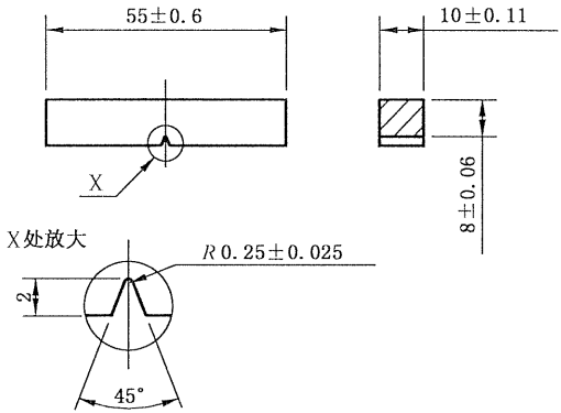
图 6 冲击试样
