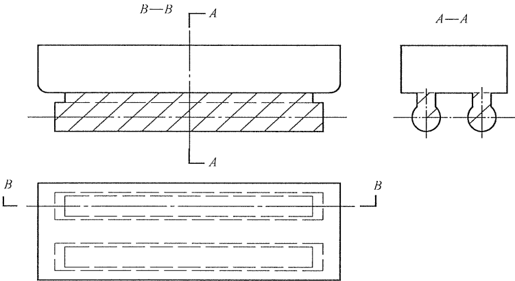
a) 试棒最小长度 L=150\text{ mm}
