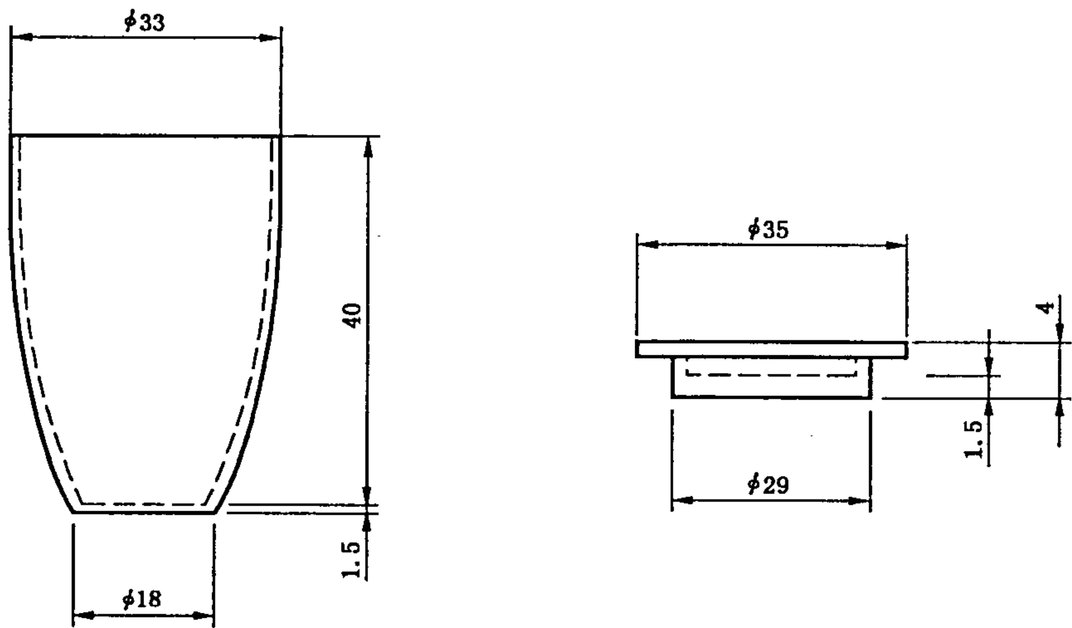
图 3 挥发分坩埚
