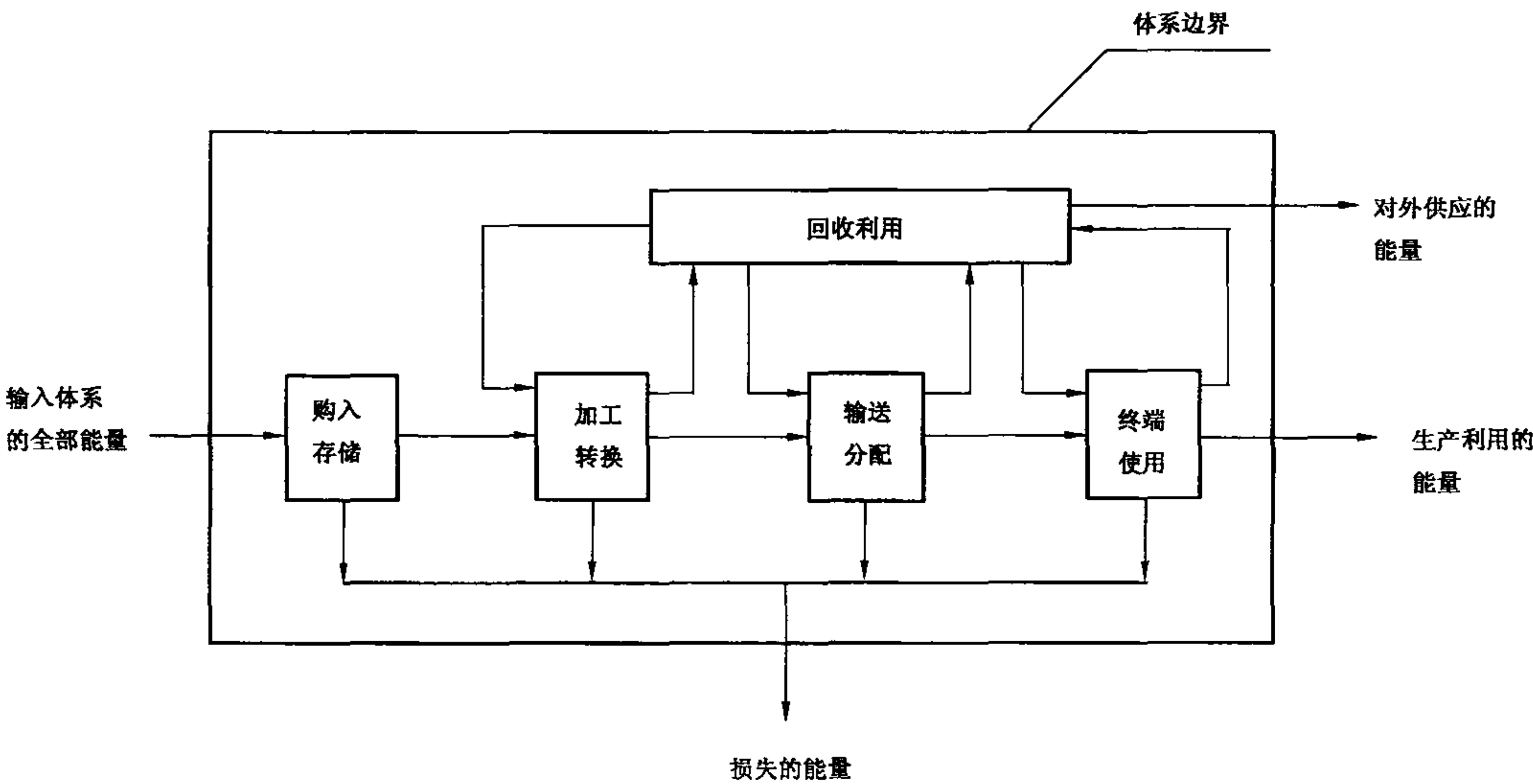
图 1 企业能量平衡框图
